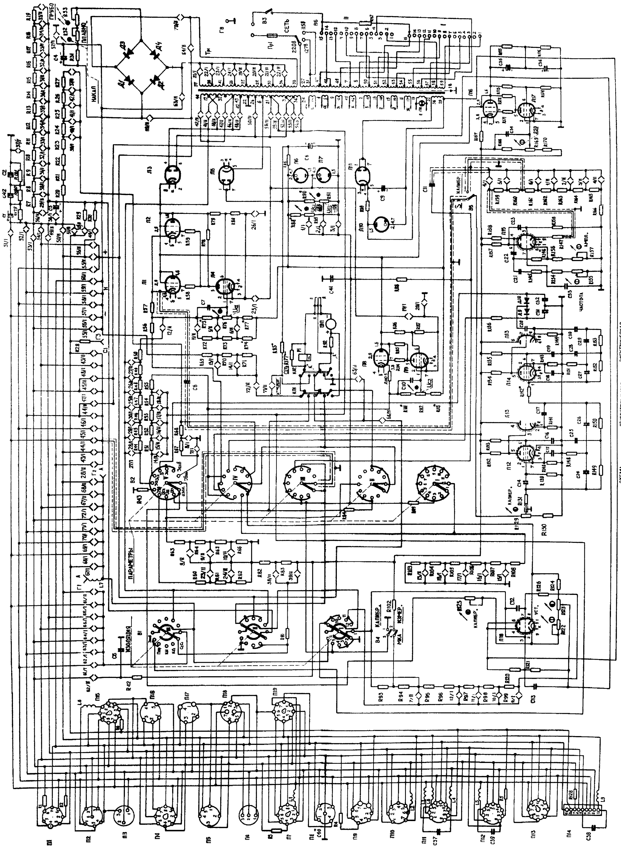
СХЕМА ЭЛЕКТРИЧЕСКАЯ
